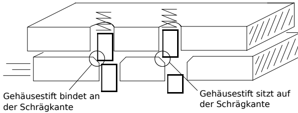
Abbildung 9.6: Der Gehäusestift klemmt in der Schrägläche
